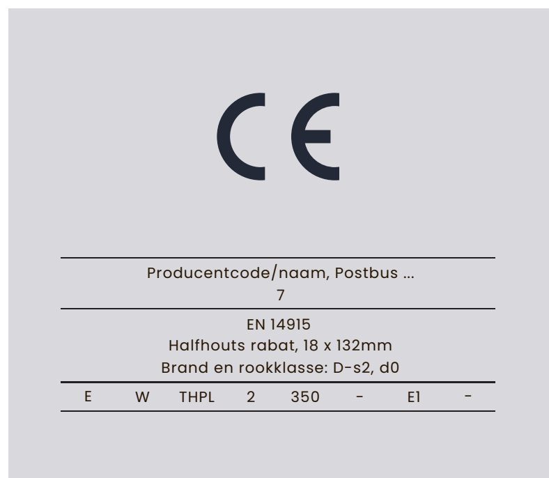
Figuur 1 voorbeeld verkorte CE-markering voor gevelbekledingen van hout.
